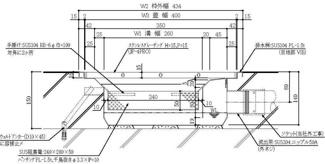
(JP-HMK-350)+(JP-4PRO) 排水柵 (A - A) 断面詳細図 S=1/3
